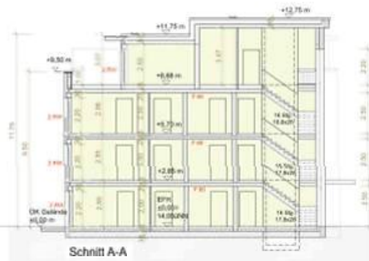
Schnitt A-A
