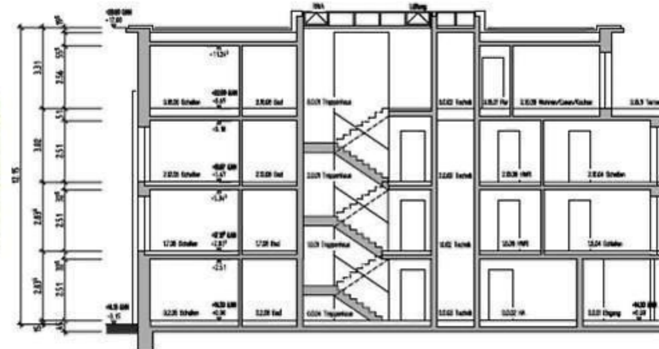
SCHNITT A-A
