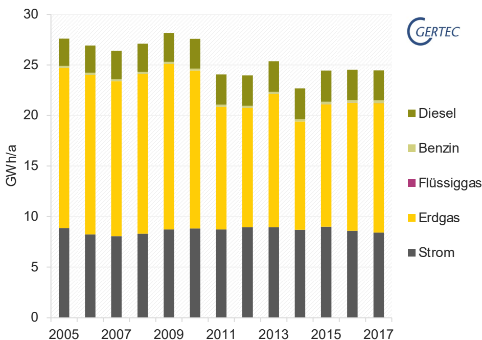
Abbildung 6 Endenergieverbrauch der Stadtverwaltung Kleve (Quelle: Gertec)
