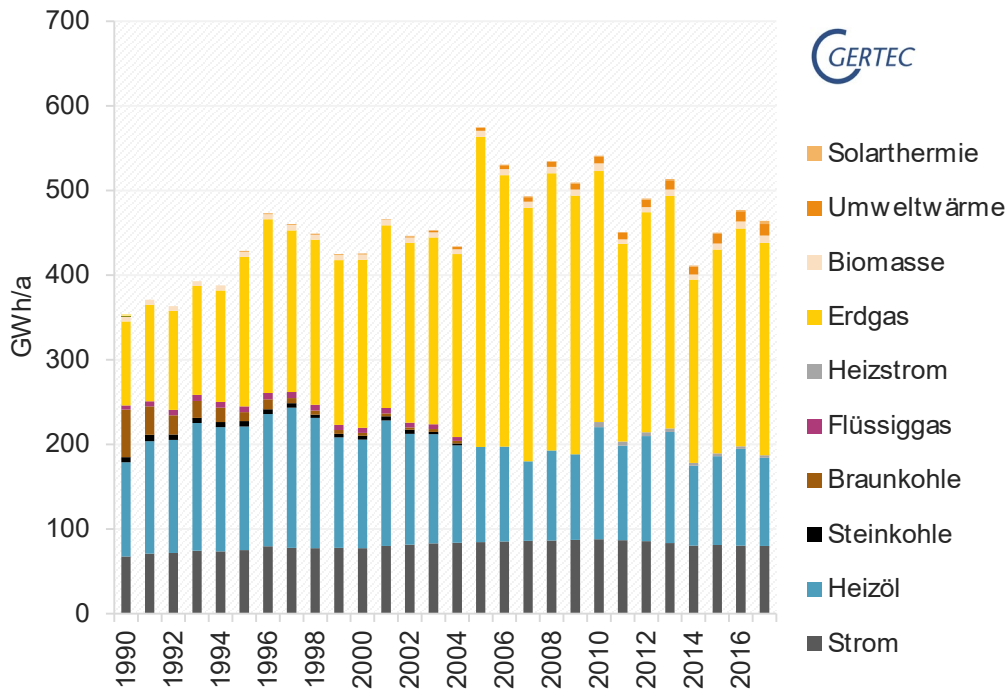
Abbildung 3 Endenergieverbrauch der privaten Haushalte in Kleve (Quelle: Gertec)
