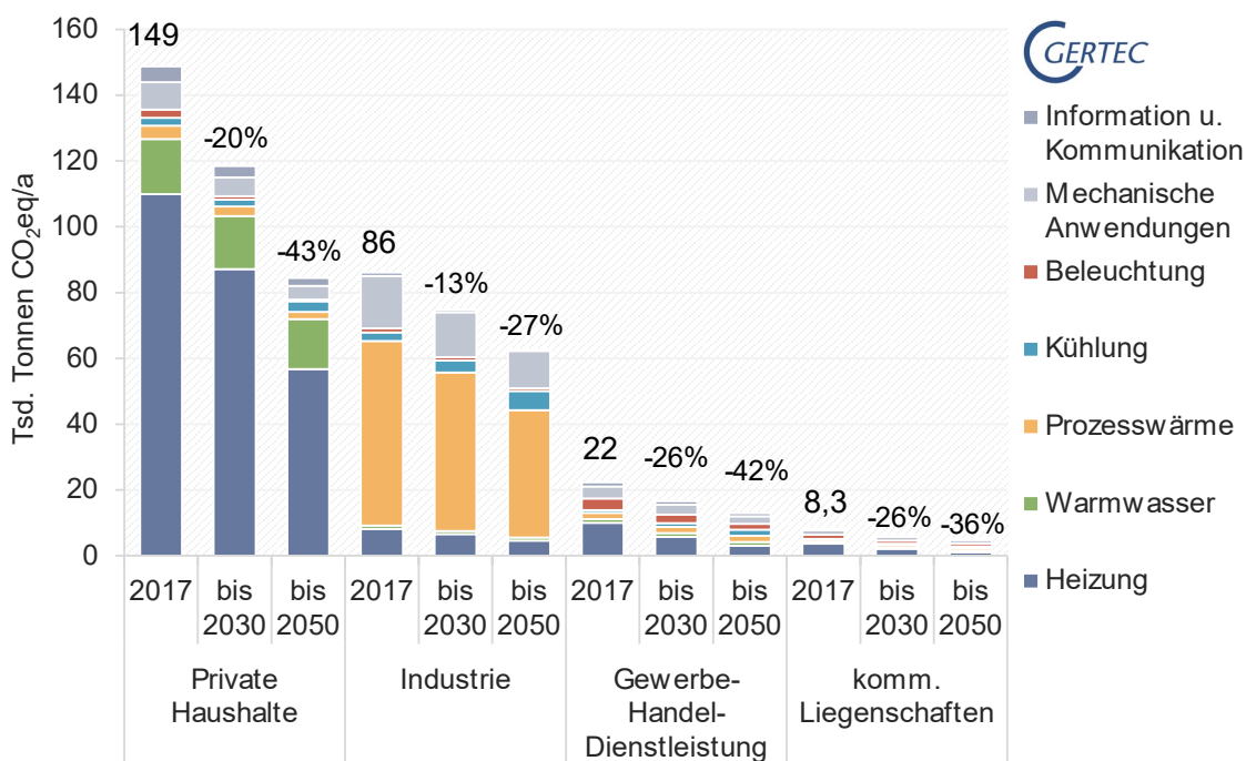
Abbildung 15 THG-Einsparpotenziale nach Sektoren und Anwendungszwecken (Quelle: Gerotec)
