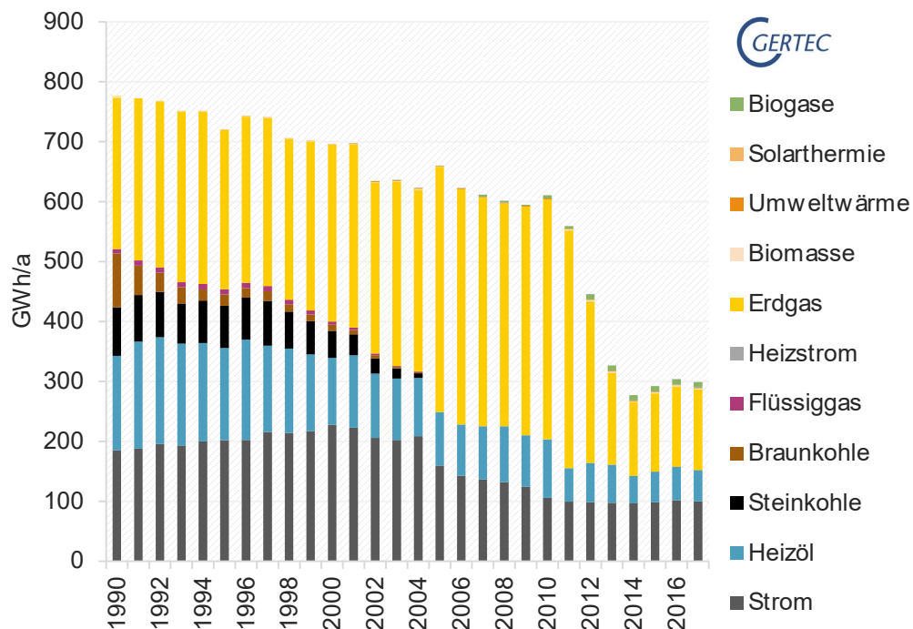
Abbildung 4 Endenergieverbrauch der Wirtschaft in Kleve (Quelle: Gertec)
