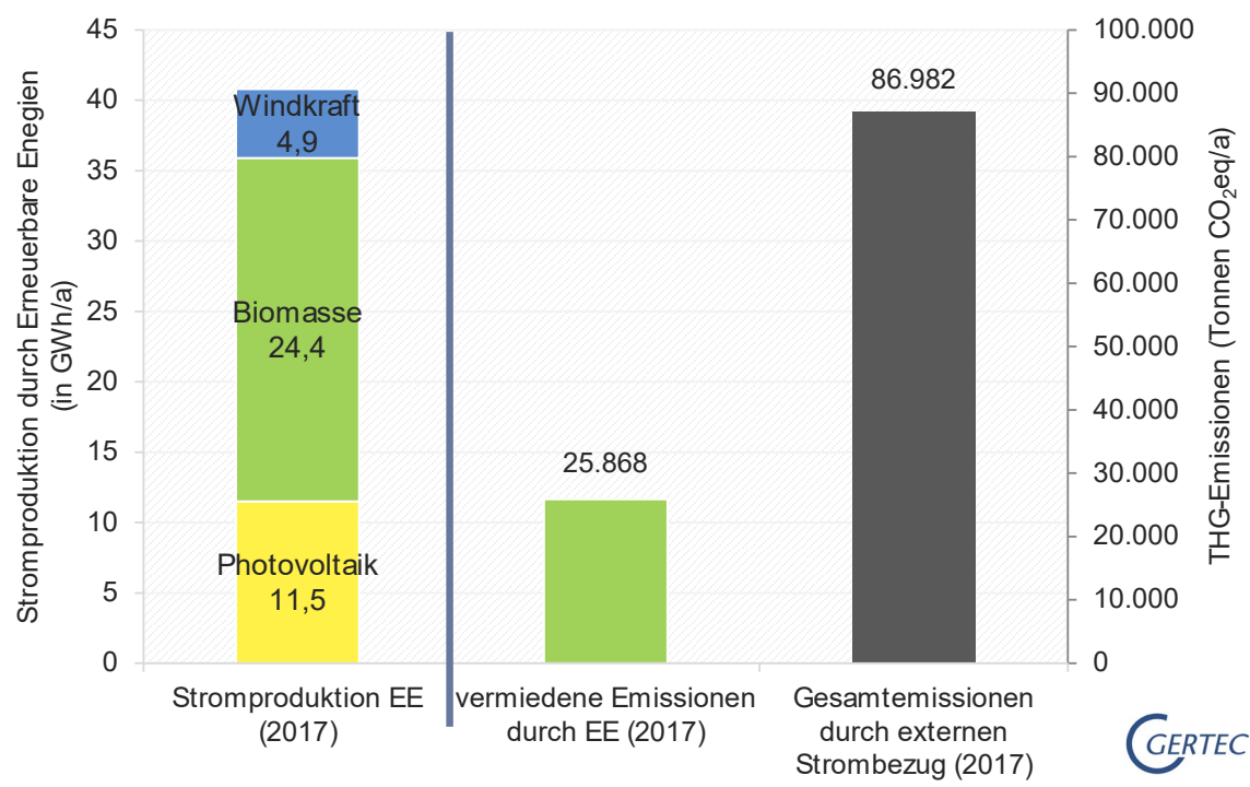
Abbildung 11 Lokale Stromproduktion in Kleve durch Erneuerbare Energien sowie hierdurch vermiedene THG-Emissionen (2017) (Quelle: Gertec)
