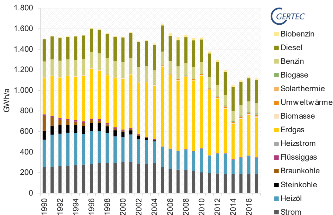
Abbildung 2 Endenergieverbrauch in Kleve 1990 bis 2017 (Quelle: Gertec)
