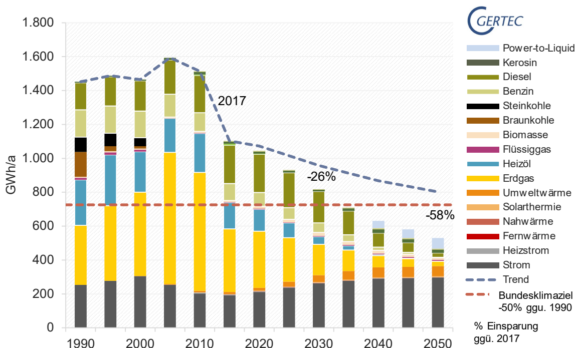
Abbildung 24 Klimaschutzszenario 95: Endenergieverbrauch nach Energieträgern – Ausschöpfung der technisch-wirtschaftlichen Potenziale bis 2050 (grafisch) (Quelle: Gertec).
