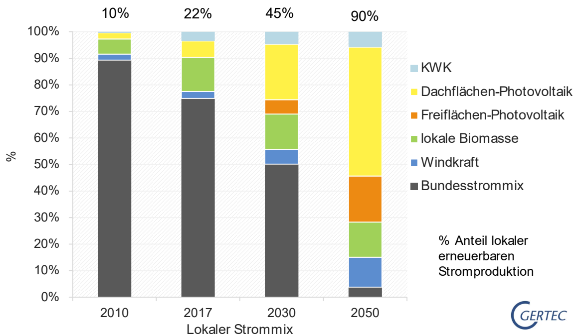
Abbildung 21 Lokaler Strommix in Kleve für die Jahre 2010 und 2017, sowie der prognostizierte lokaler Strommix für 2030 und 2050 (grafisch) (Quelle: Gertec)
