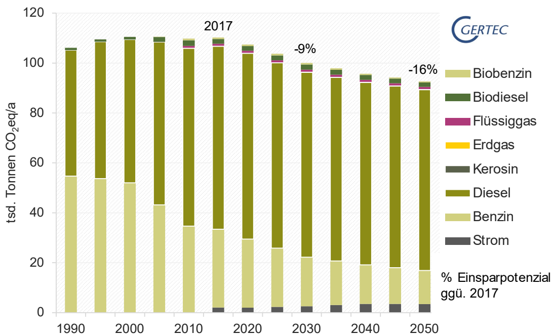
Abbildung 18 THG-Emissionen nach Trendszenario des BMU – übertragen auf die Stadt Kleve (1990 – 2050) (Quelle: Gertec).
