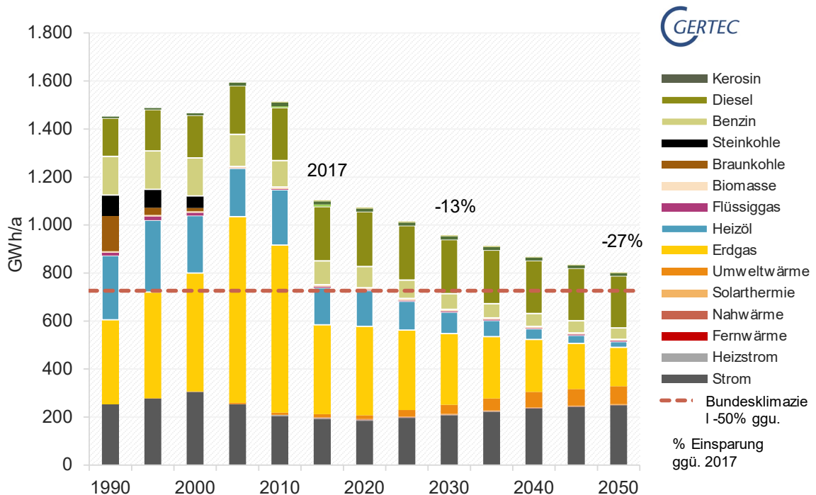
Abbildung 22 Trendszenario – Endenergieverbrauch nach Energieträgern bis 2050 (grafisch) (Quelle: Gertec)
