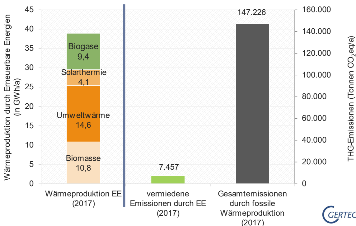
Abbildung 12 Lokale Wärmeproduktion in Kleve durch Erneuerbare Energien sowie hierdurch vermiedene THG-Emissionen (2017) (Quelle: Gertec)
