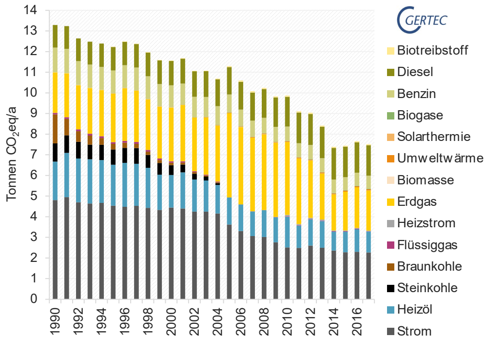
Abbildung 10 THG-Emissionen je Einwohner in Kleve (Quelle: Gertec)
