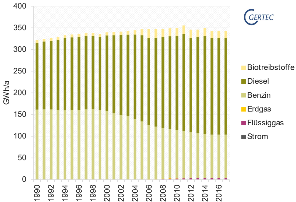
Abbildung 5 Endenergieverbrauch im Verkehrssektor in Kleve (Quelle: Gertec)
