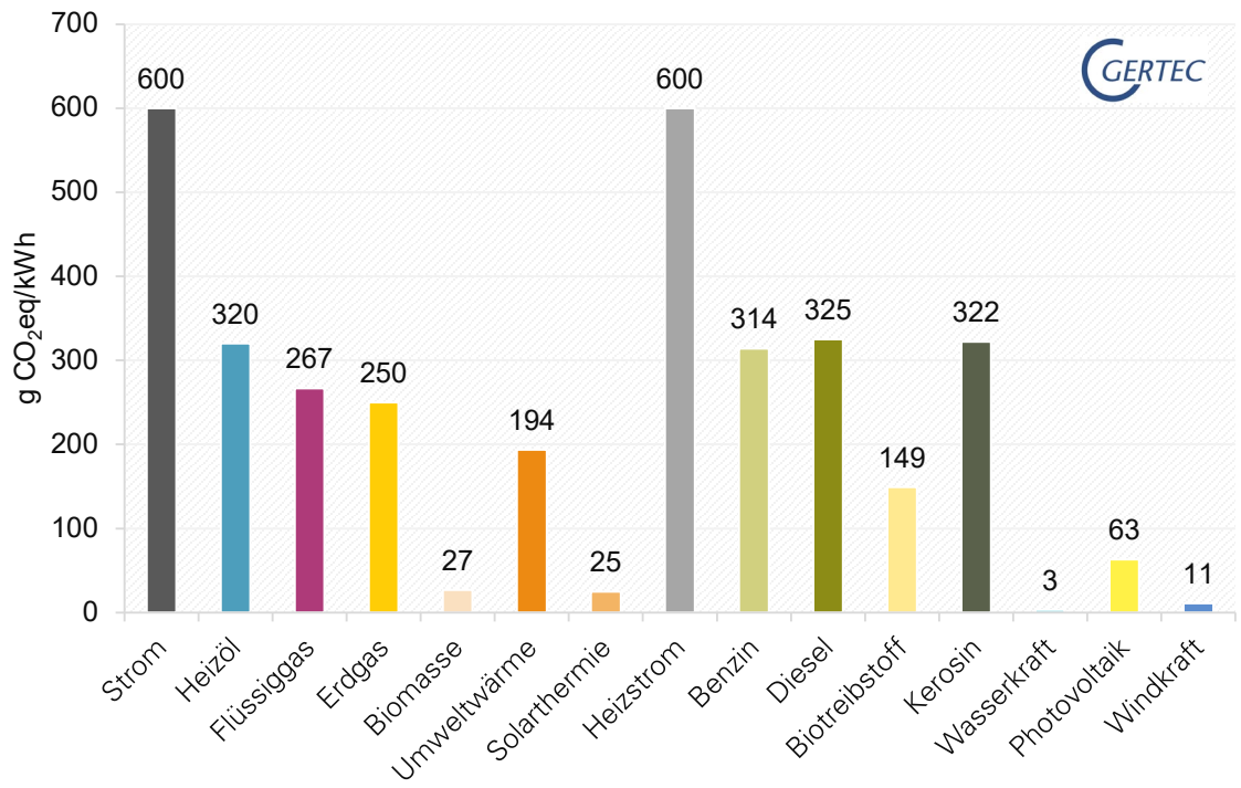
Abbildung 1 Für Kleve relevante Emissionsfaktoren im Jahr 2017 (Quelle: Gertec nach Daten aus ECOSPEED Region smart )
