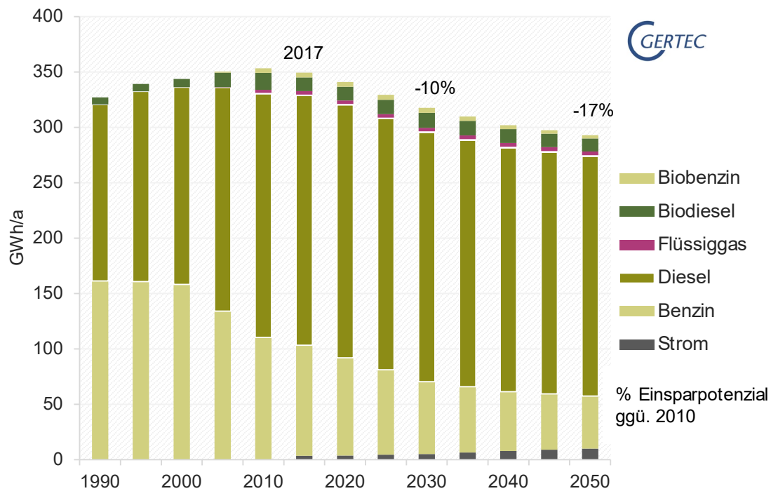
Abbildung 16. Energieverbräuche nach Trendszenario des BMU – übertragen auf die Stadt Kleve (1990 – 2050) (Quelle: Gertec).
