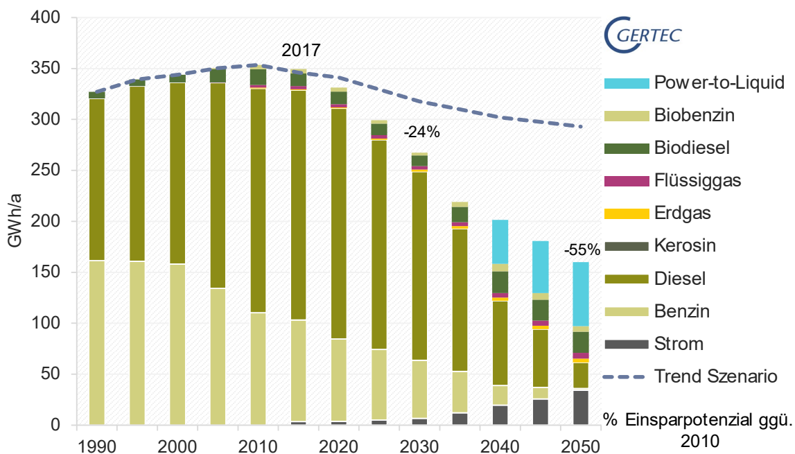
Abbildung 17 Energieverbräuche nach Klimaschutzszenario des BMU – übertragen auf die Stadt Kleve (1990 – 2050) (Quelle: Gertec).
