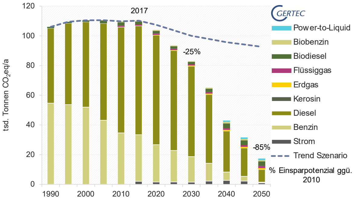
Abbildung 19 Potenzial der THG-Emissionsminderung in Kleve bis 2050 auf Basis des Klimaschutzszenarios des BMU (Quelle: Gertec).
