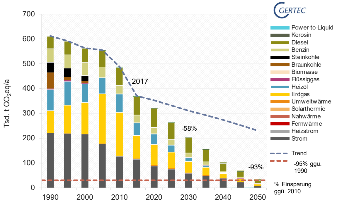
Abbildung 25 Klimaschutzszenario 95: THG-Emissionen nach Energieträgern (grafisch); (Quelle: Gertec)
